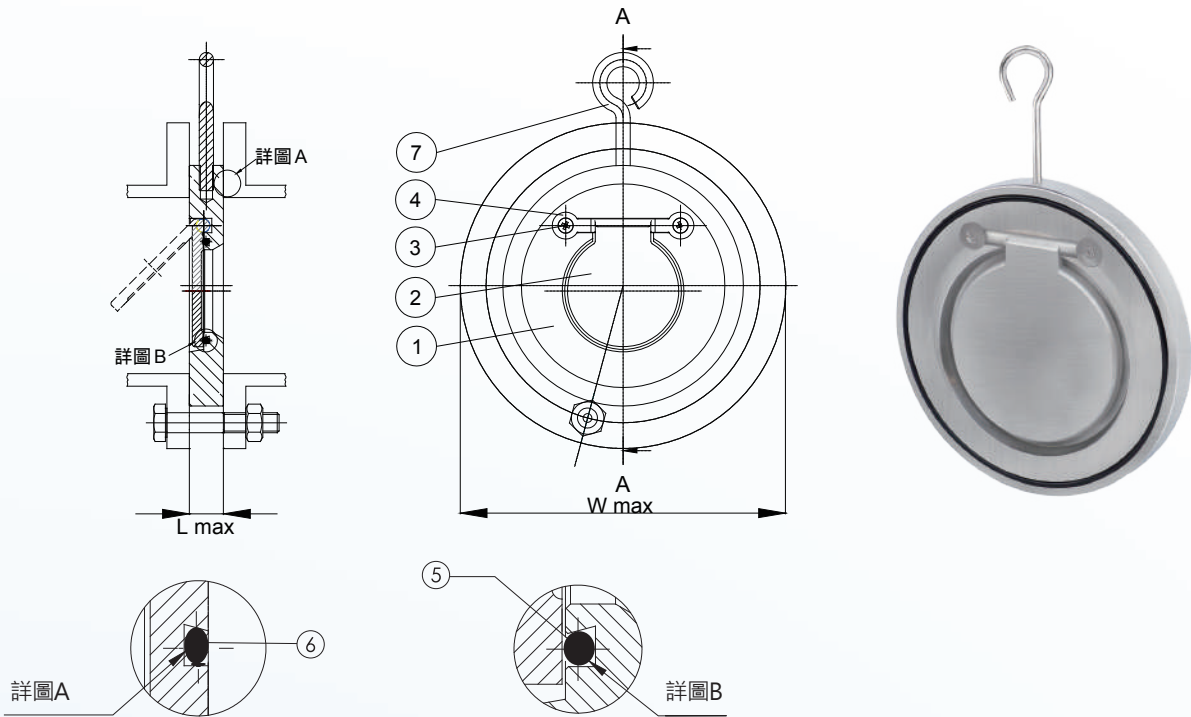
DIMENSION 尺寸表
