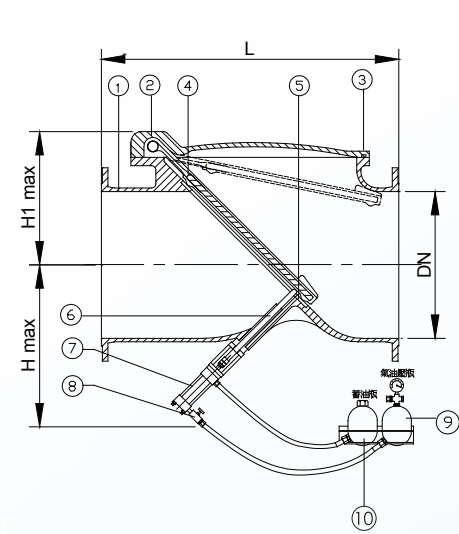
DIMENSION 尺寸表
