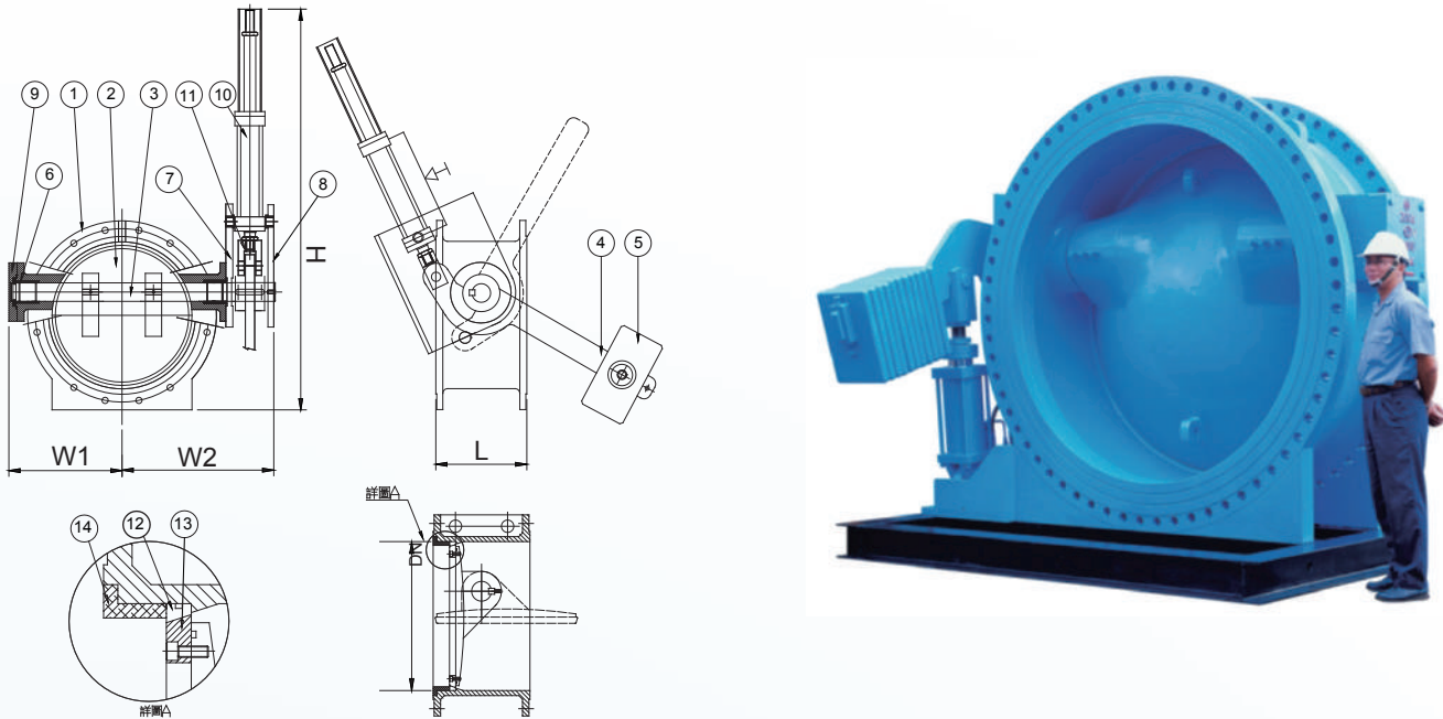
DIMENSION 尺寸表
