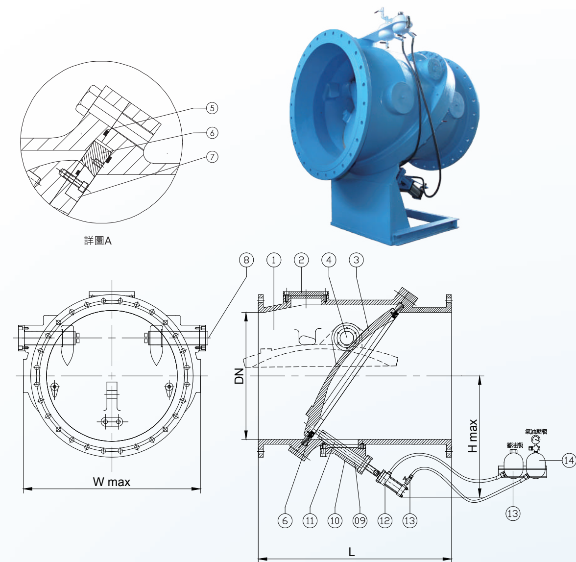
DIMENSION 尺寸表
