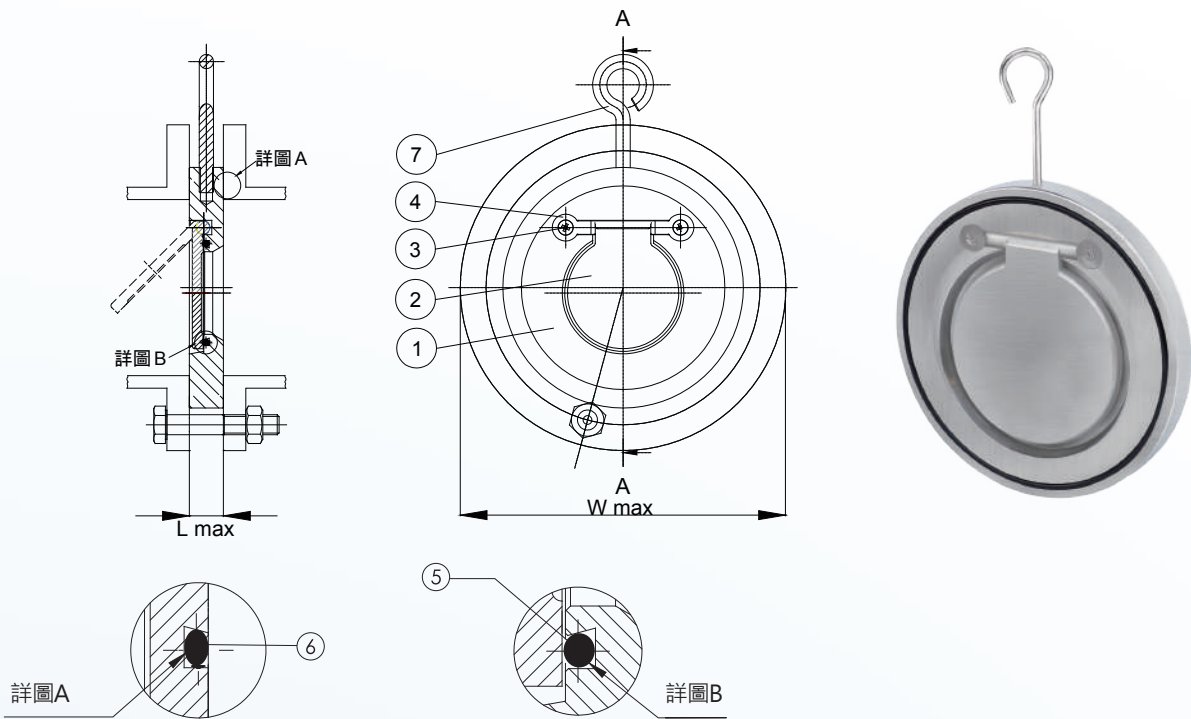
DIMENSION 尺寸表
